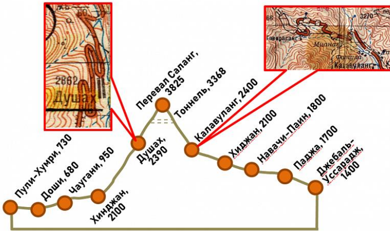
Схема профиля тоннеля Саланг/ © russiancouncil.ru
