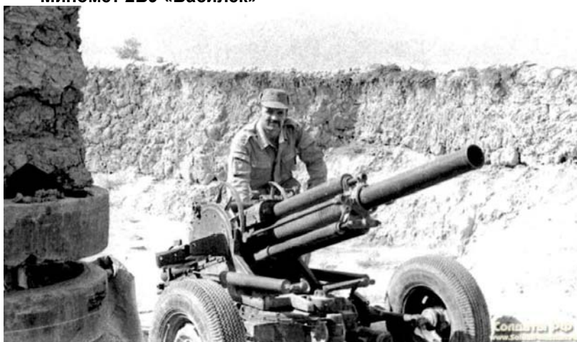
Миномёт 2Б9 «Василек»
